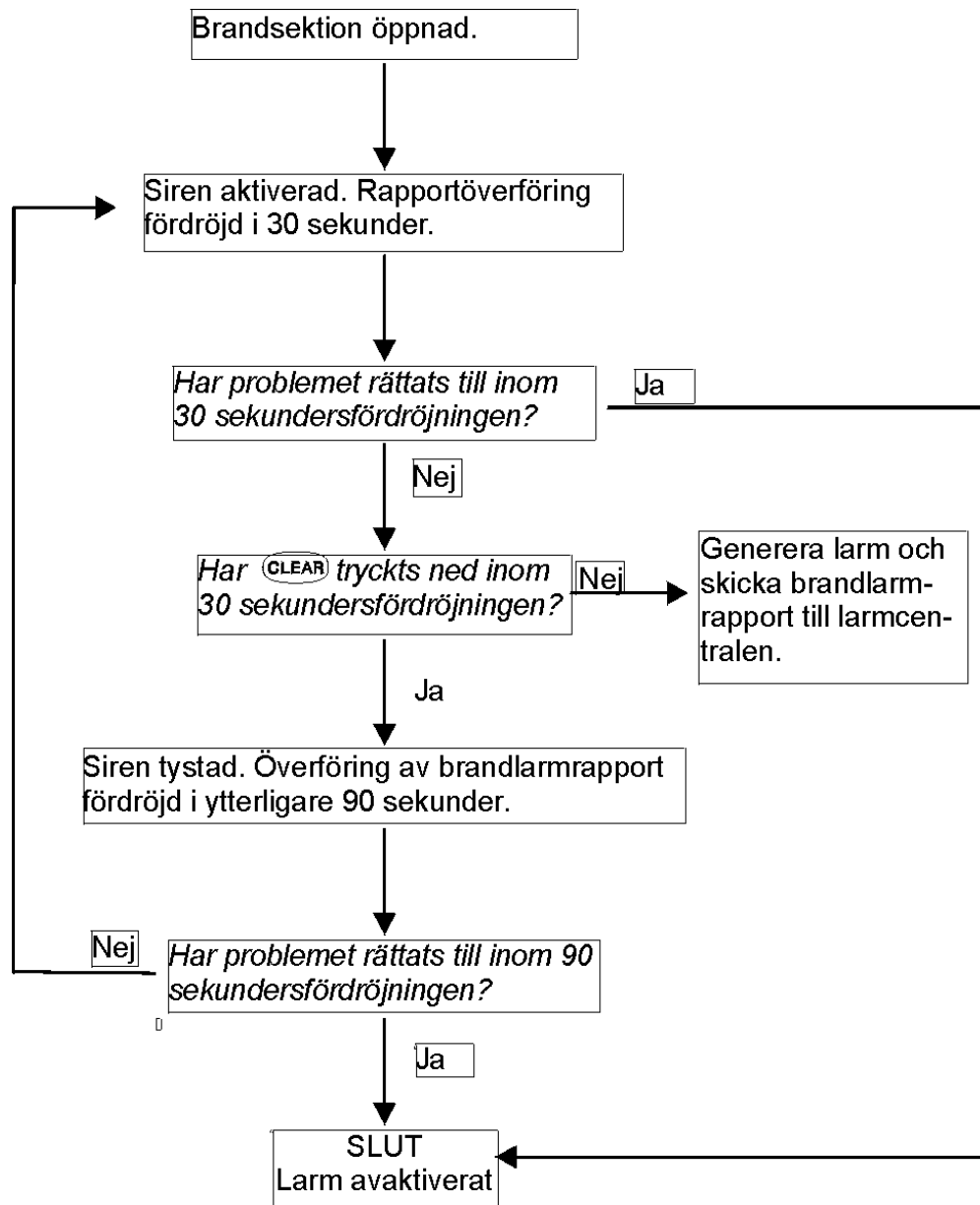
Figur 6.1: Fördröjd brandsektion – händelsesekvens
