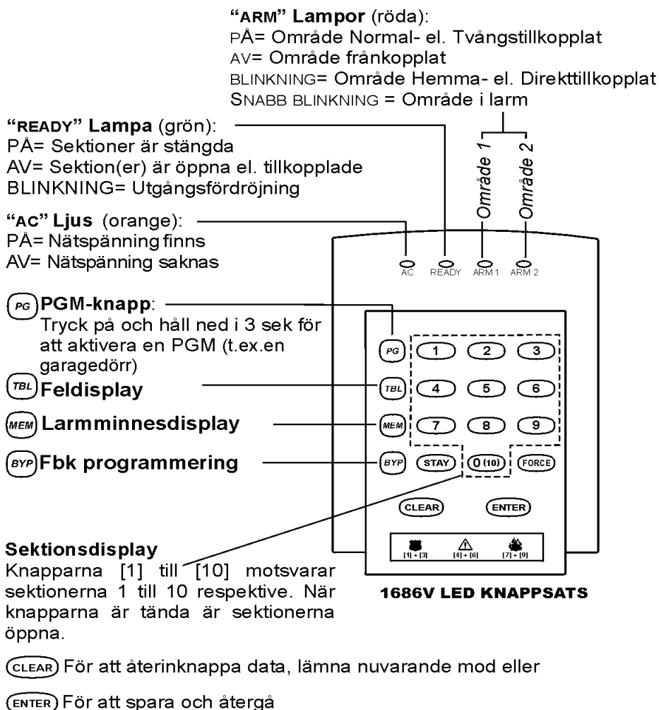
Figur 2.1: Översikt av 1686V LED Knappsatsen
